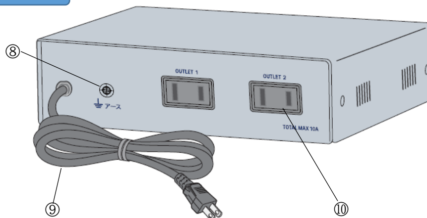
リアパネル
